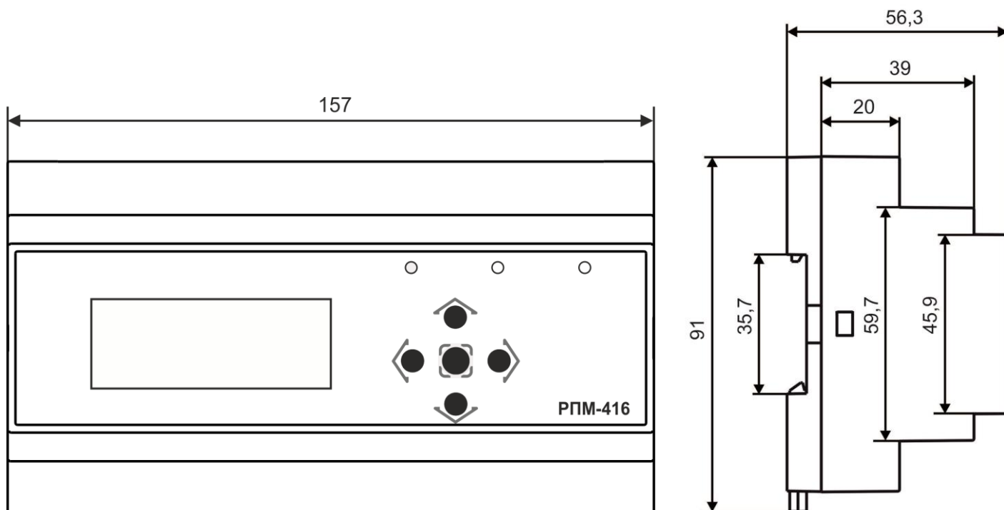
Рисунок 1.1 – Внешний вид и габаритные размеры регистратора
