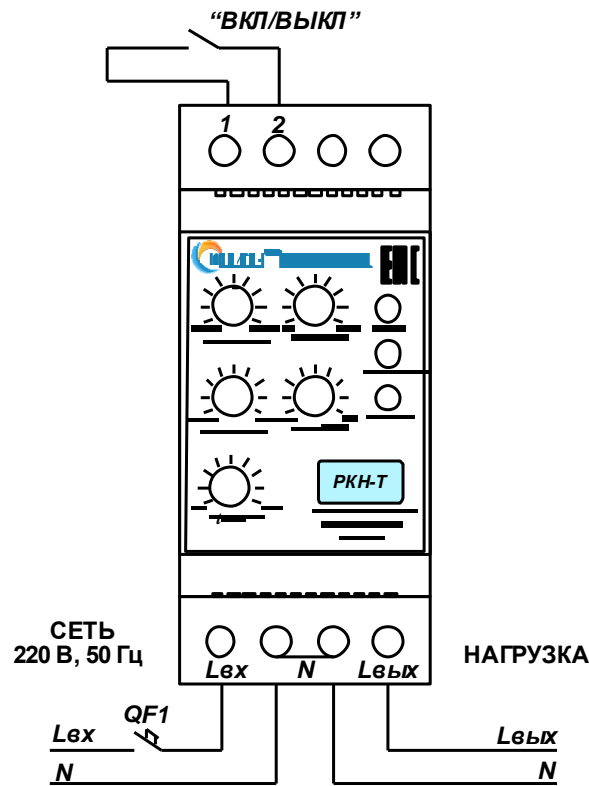
Рис.1. Порядок подключения реле.
