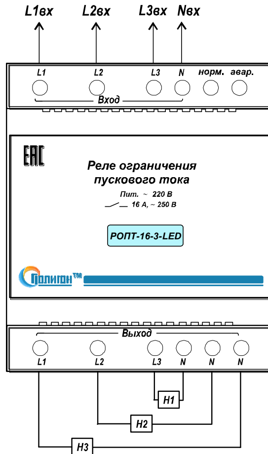
Рис.1. Типовая схема подключения РОПТ-16-3-LED.
